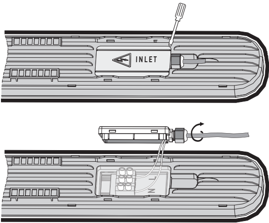
Рис.2 Подключение светильника PWP-C5 PRO
